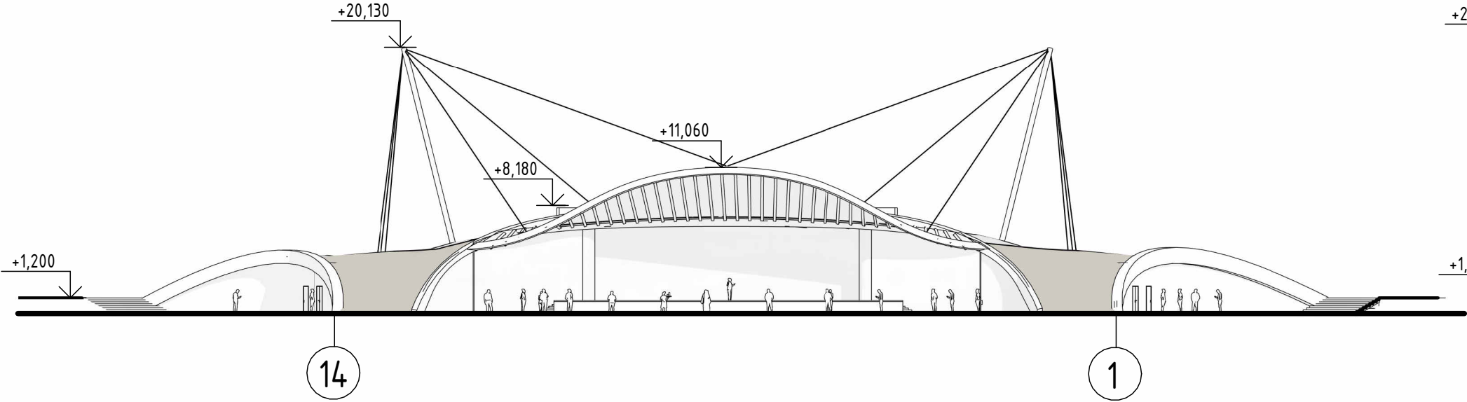
ФАСАД В ОСЯХ 1-14
