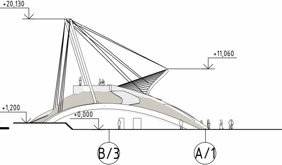
РАЗРЕЗ 1-1
